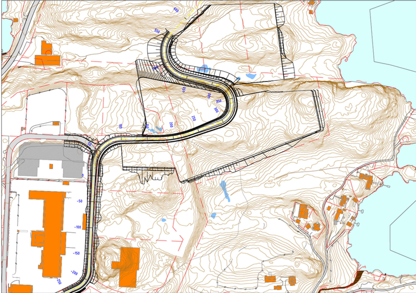
Figur 19 Plantegning med mulig vegløsning og utvidelse av næringsområdet nordover
