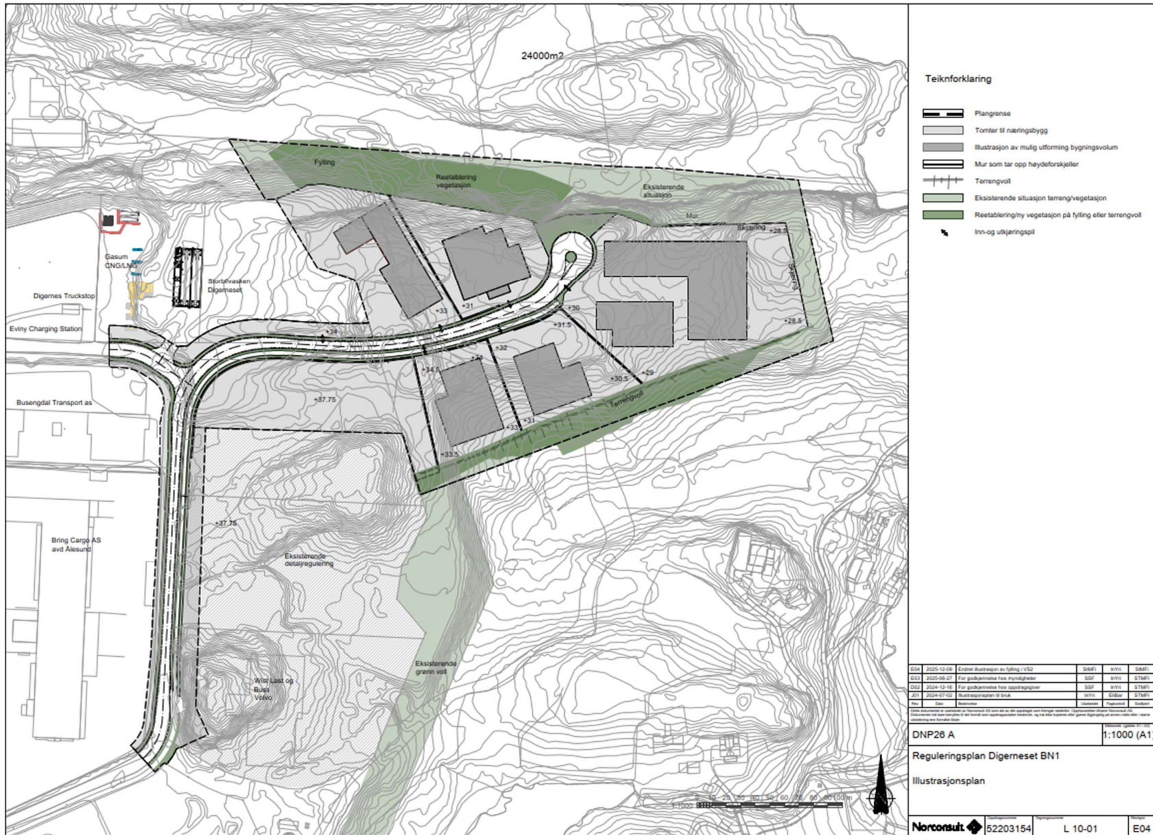
Figur 2 illustrasjonsplan
