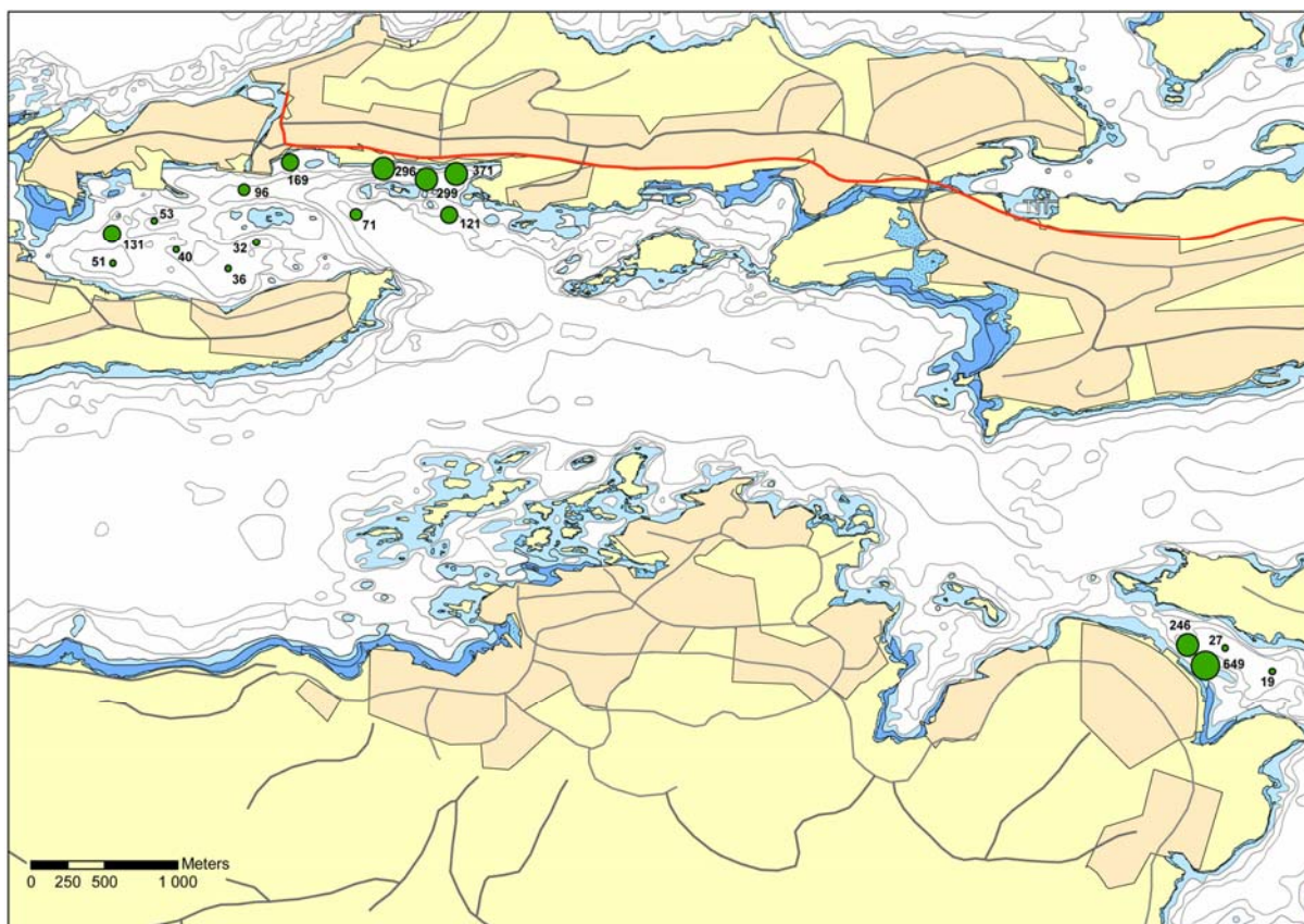
Figur 6. Beregnet risiko for økologien ( C_{sed} / MPC ) på de enkelte stasjonene i henhold til trinn 2. Tallet over symbolene angir antall ganger den totale risikoen ( C_{sed} ) overskrider grenseverdien for de forskjellige stoffene. Størrelsen på symbolene illustrerer størrelsen på risikobidraget.
