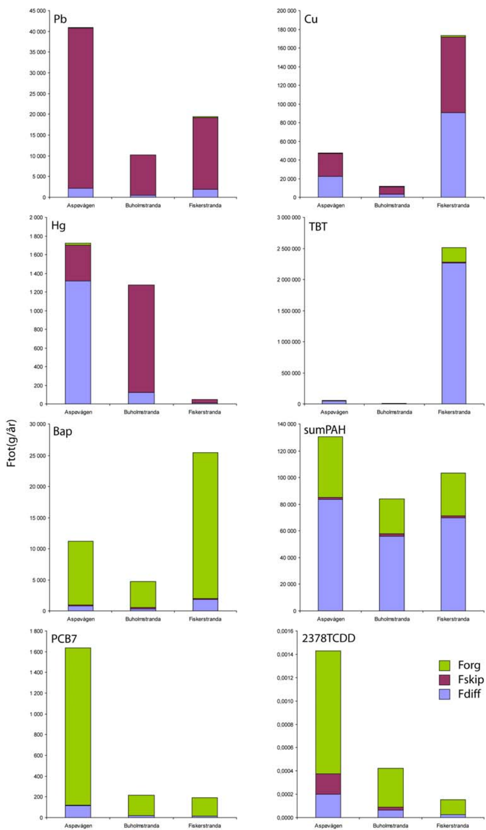
Figur 3. Beregnet total spredning (g/år) for de tre delområdene ved diffusjon ( F_{diff} ), skipsoppvirvling ( F_{skip} ) og via organismer ( F_{org} ).
